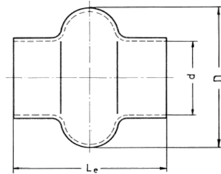
I: für Einfachgelenke ( mit einem Balg)
